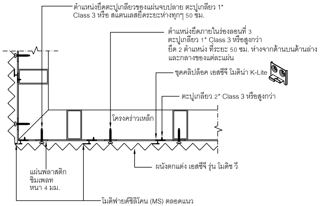
Detail ผนังงานบริเวณมุงนอก
