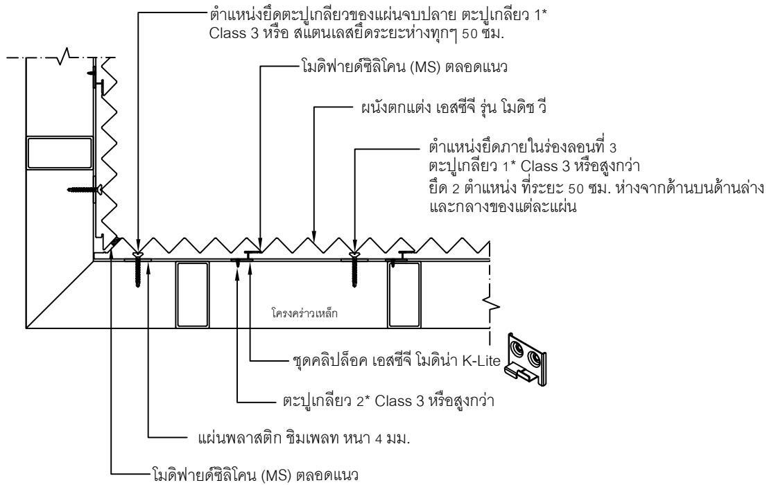
Detail ผนังงานบริเวณมุงใน
