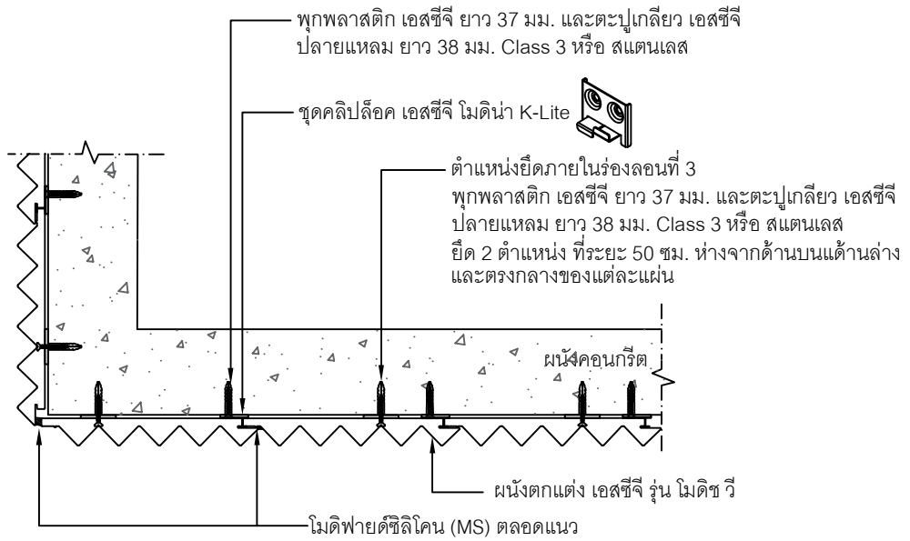
Detail ใช้งานบริเวณมุงนอก
