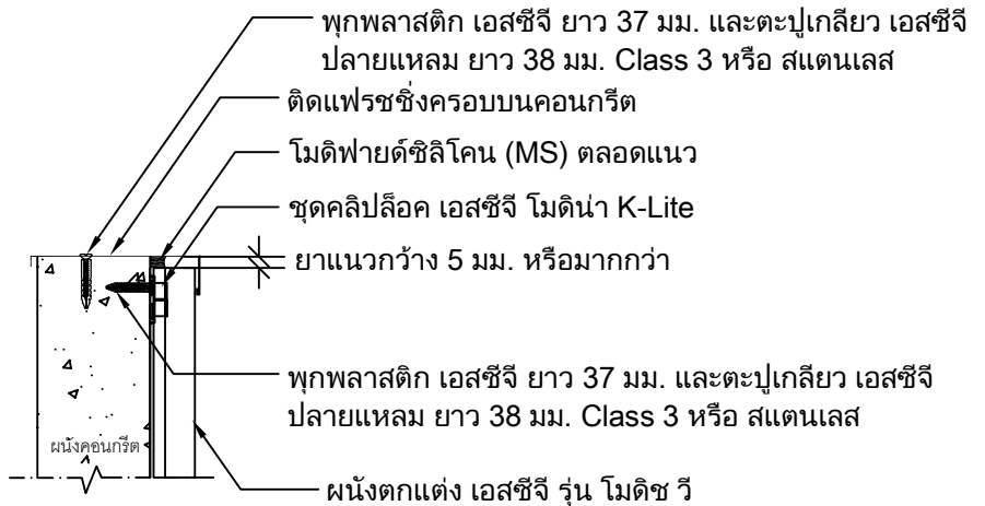
Detail งบประมาณด้านบน (กรณีผนังภายนอก)
