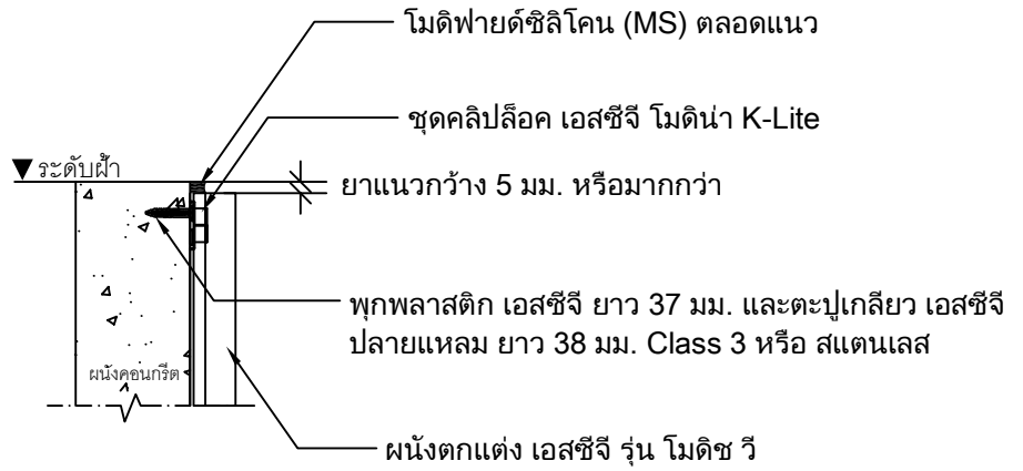
Detail งบประมาณด้านบน (กรณีผนังภายใน)
