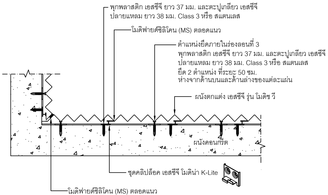
Detail ใช้งานบริเวณมุงใน
