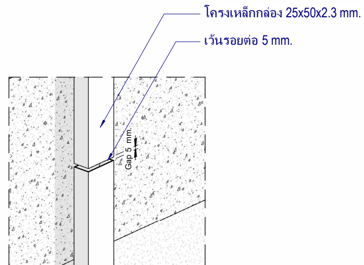
แบบขยาย Left View
