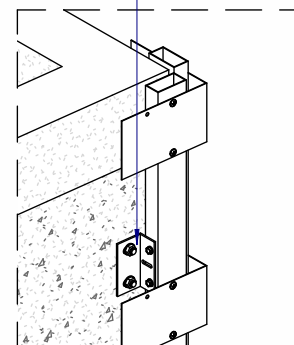
แบบขยาย Left View
