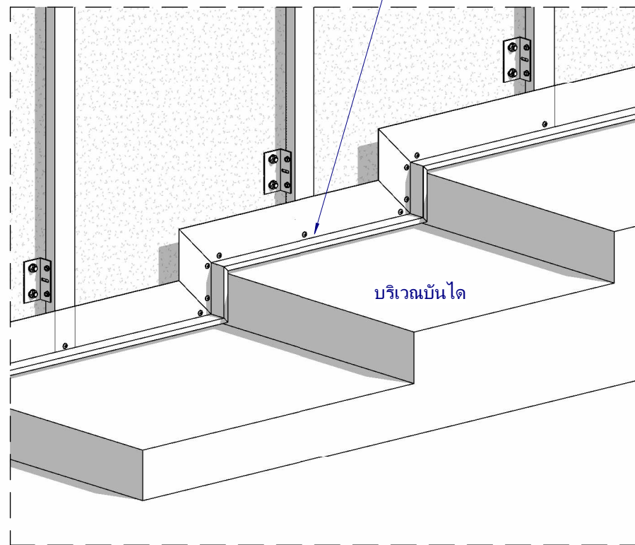
3D View การติด Flasing เข้ากับโครง เหล็ก Section หน้าที่ A07
