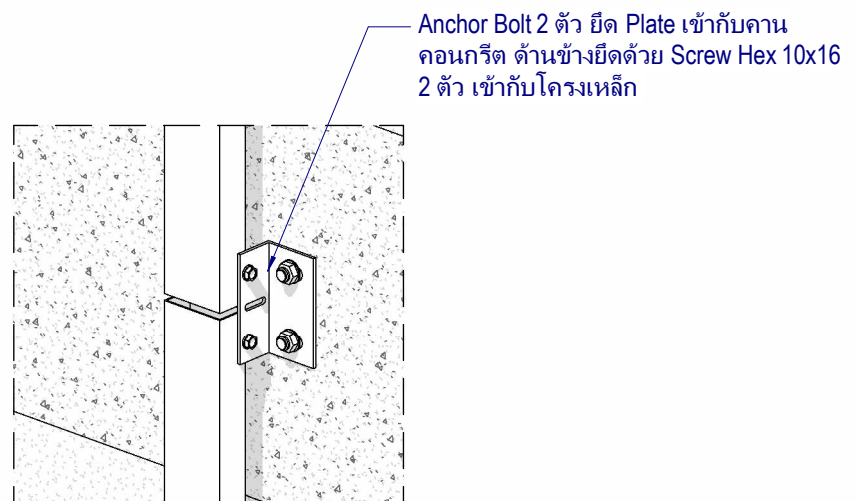
แบบขยาย Right View
