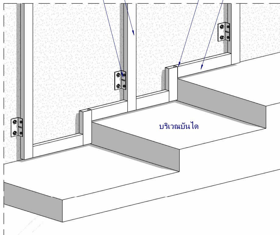
3D View การติดโครงเหล็ก และเหล็ก เสริมสำหรับรับ Flasing
