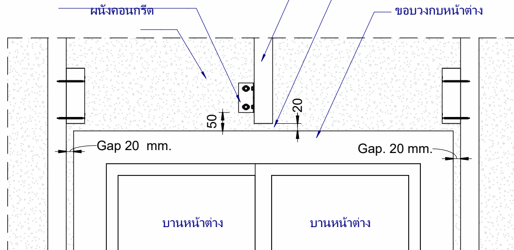
แบบขยาย A
