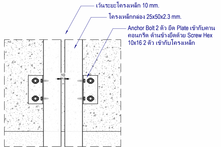
แบบขยาย Front View
