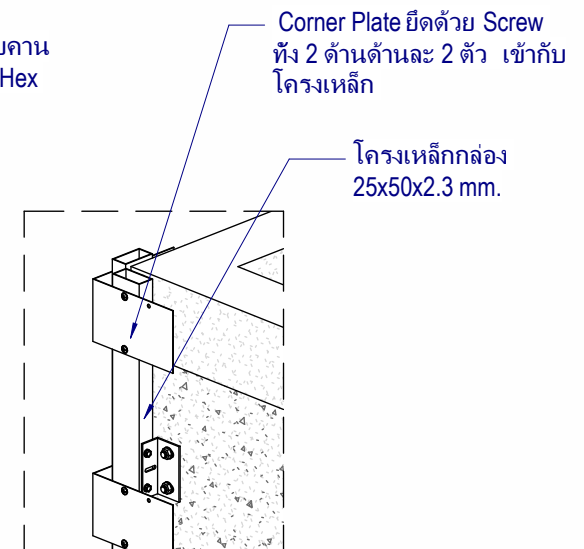
แบบขยาย Right View
