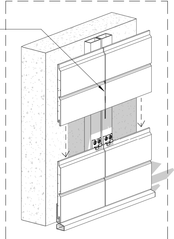
3D View การเรียงแผ่นในแนวตั้ง กรณี รอยต่อแผ่นเว้นร่องยาแนว
