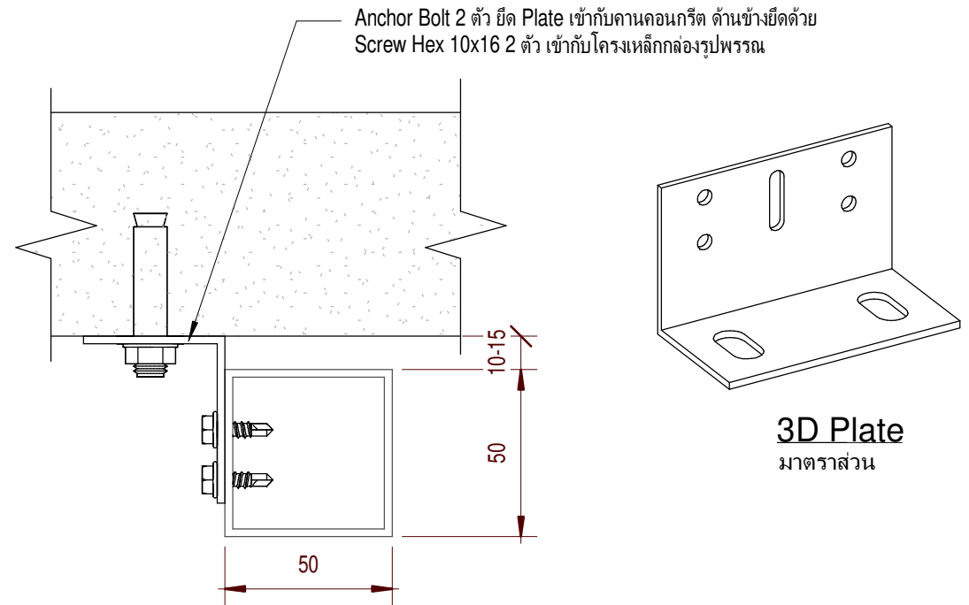
Detail การยึด Plate เข้ากับโครงเหล็ก มาตราส่วน 1 : 2
