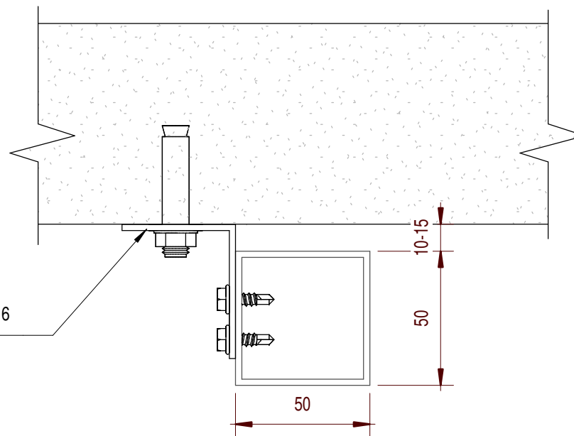
Detail การยึด Bracket เข้ากับโครงเหล็ก มาตราส่วน 1 : 2
