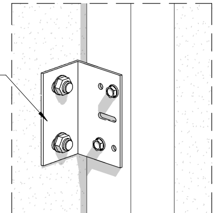
3D Detail การยึด Plate เข้ากับโครงเหล็ก มาตราส่วน
