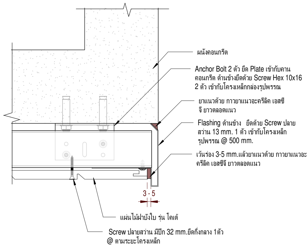
Detail การจบงานด้วย Flashing ด้านข้าง
