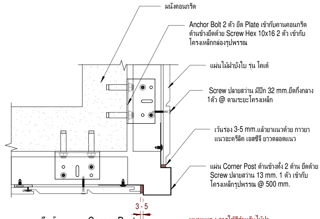
กรณี เข้ามุมแบบ Corner Post
