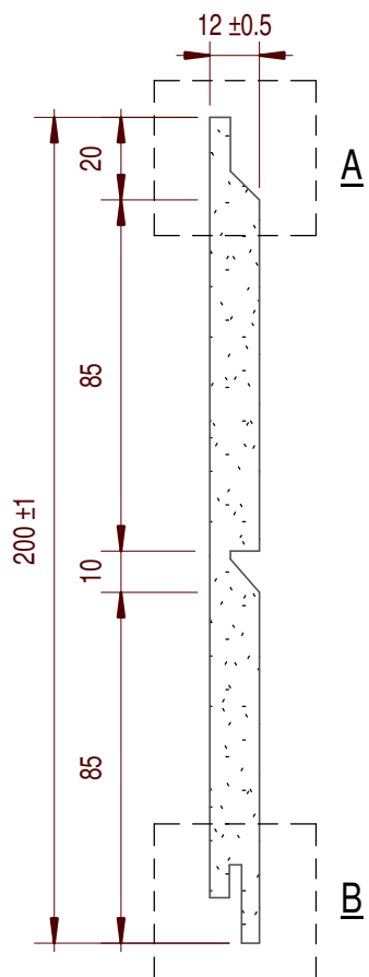
Section มาตราส่วน 1 : 2
