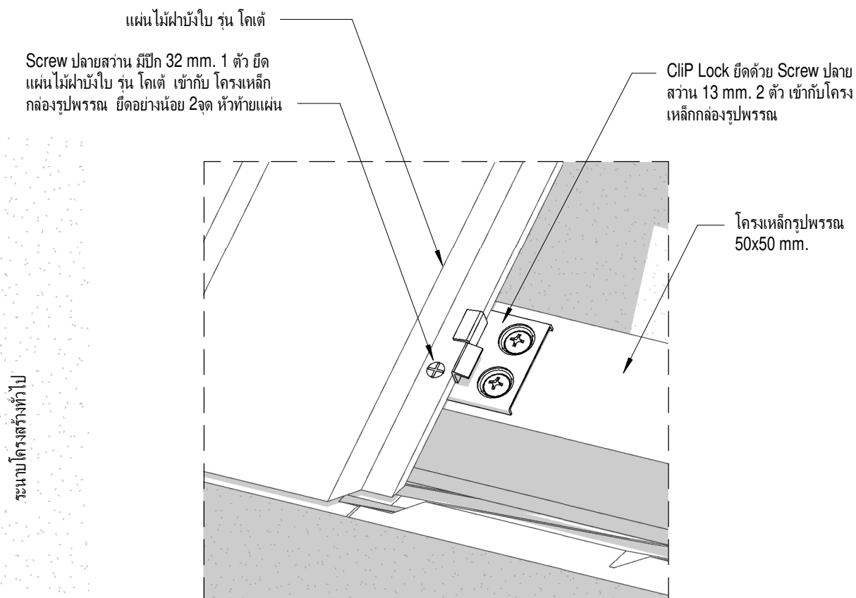
แบบขยาย การยึดแผ่นเข้ากับโครงเหล็ก 3D View
