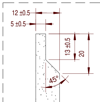
แบบขยาย A มาตราส่วน 1 : 1
