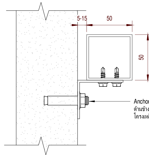
Detail-1 การยึด Plate เข้ากับโครงเหล็ก มาตรฐาน 1 : 2
