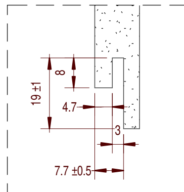
แบบขยาย B มาตราส่วน 1 : 1
