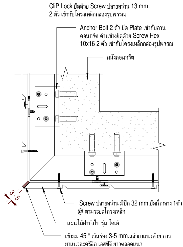
กรณี เข้ามุมแบบตัด 45°
