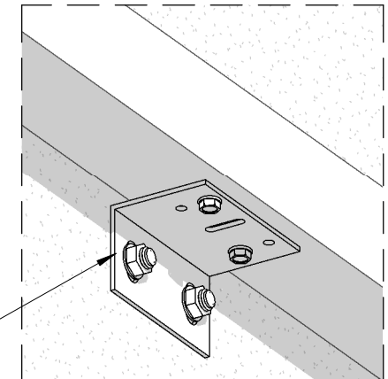
3D Detail การยึด Plate เข้ากับโครงเหล็ก มาตรฐาน
