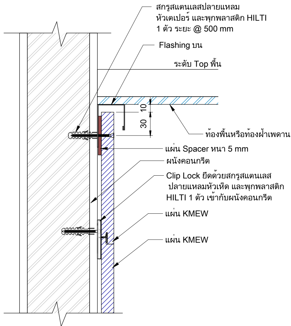
Section View - กรณีแผ่น KMEW จบงานด้วย Flashing บน
