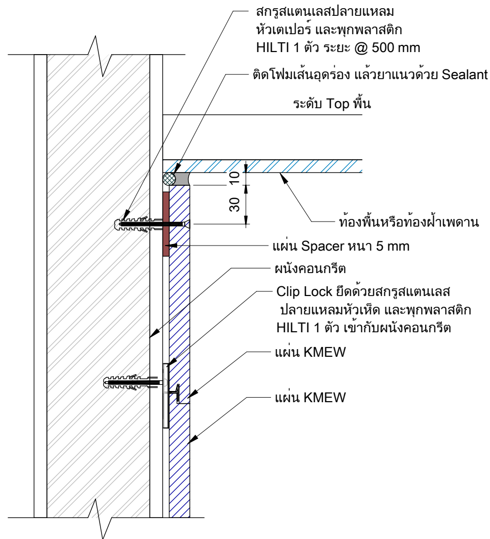
Section View - กรณีแผ่น KMEW จบงานด้วย Sealant
