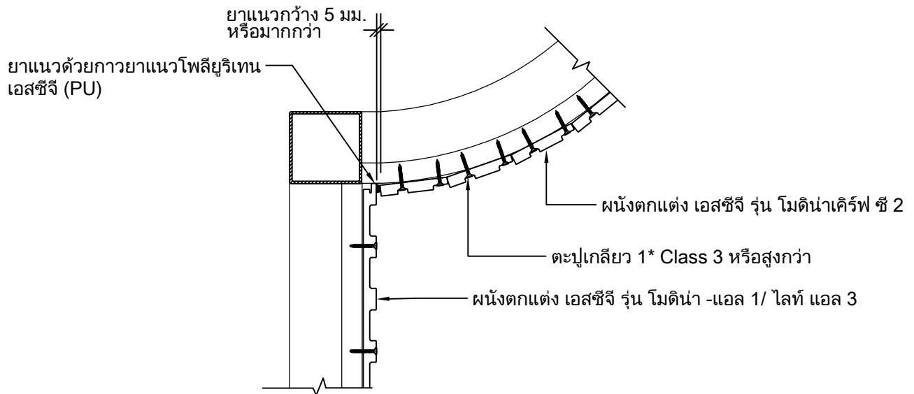
Detail จบงานด้านข้างผนังโค้งนูน กรณีชนผนังตกระตัง เอสซีจี รุ่น โมดิโน -แอล 1/ โลท์ แอล 3
