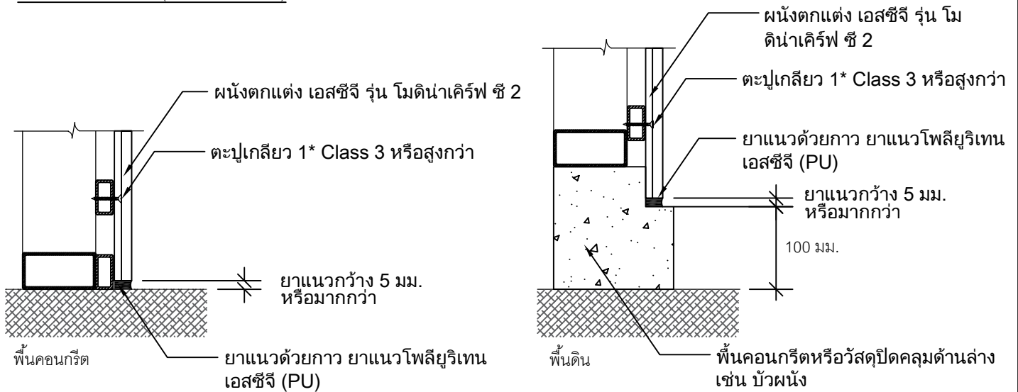
Detail 3 ผนังด้านล่าง (พื้นคอนกรีต)
