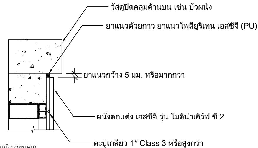
Detail 2 ผนังด้านใน (กรณีผนังภายนอก)
