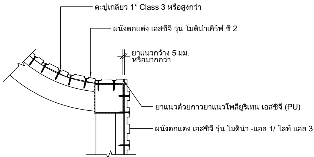
Detail จบงานด้านข้างผนังโค้งวาว กรณีชนผนังตกระตัง เอสซีจี รุ่น โมดิโน - แอล 1/ โลท์ แอล 3
