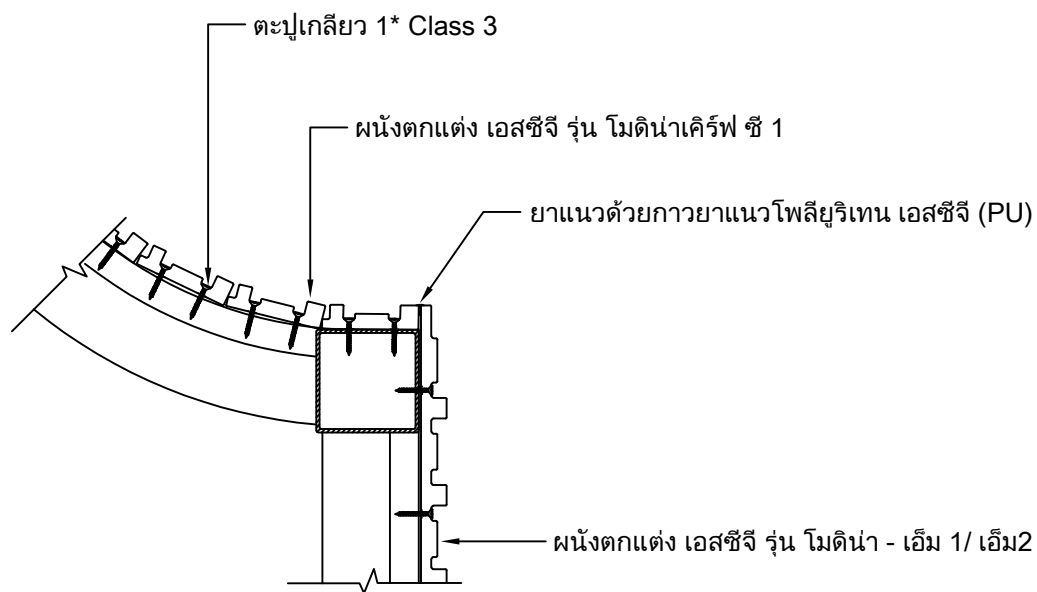
Detail งบประมาณด้านข้างผนังโค้งว้า กรณีชนผนังตกแต่ง เอสซีจี รุ่น โมดิโน - เอ็ม 1/ เอ็ม2
