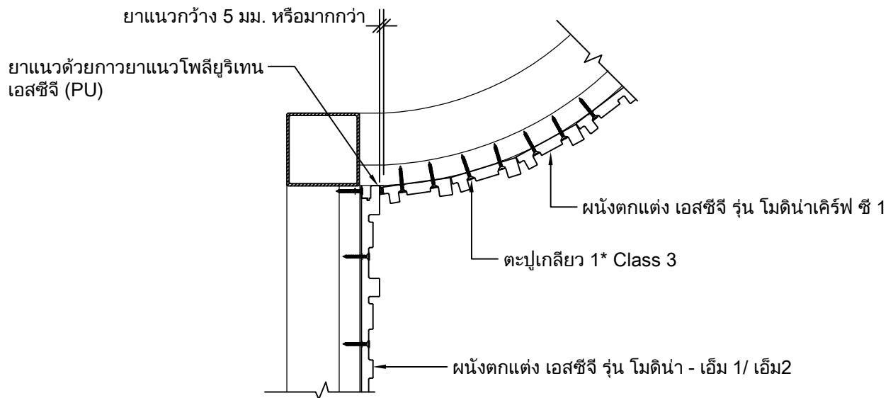
Detail งบประมาณด้านข้างผนังโค้งนูน กรณีชนผนังตกแต่ง เอสซีจี รุ่น โมดิโน - เอ็ม 1/ เอ็ม2
