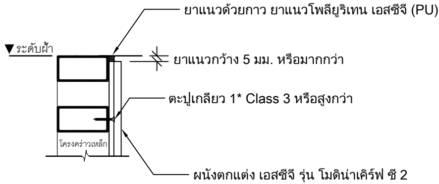
Detail 1 ผนังด้านใน (กรณีผนังภายใน)
